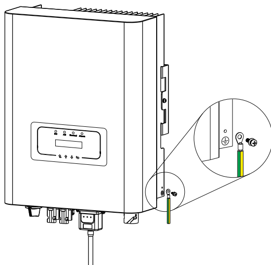
Rys. 5.11 Instalacja obudowanego przewodu uziemiającego
