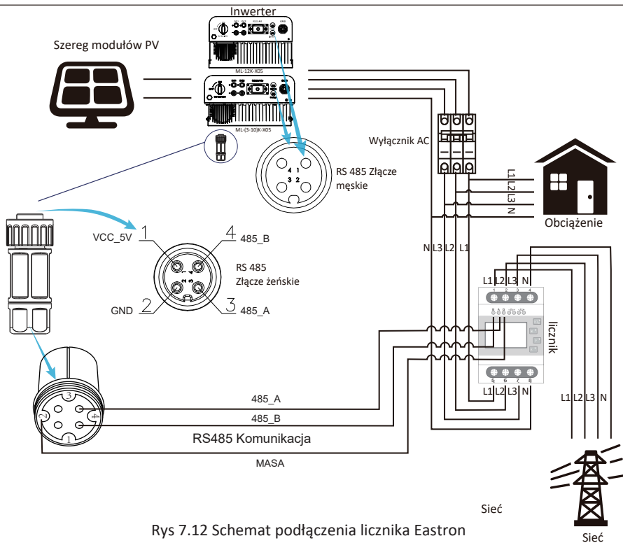
Eastron SDM630-Modbus V2
