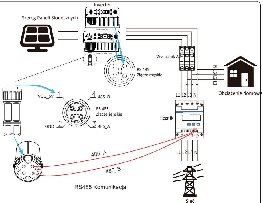
Rys 7.16 Schemat połączenia licznika CHNT
