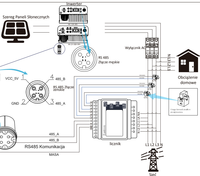
Rys. 7.14 Schemat podłączenia licznika Eastron
