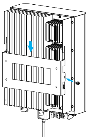
Rys. 4.6 Instalacja Inwertera
