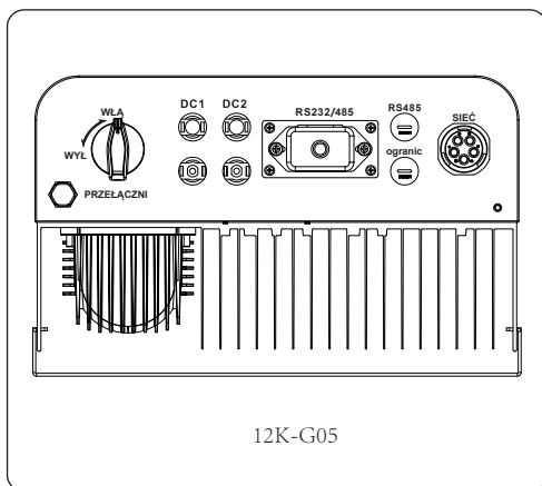
Rys. 1.2 Tył inwertera
