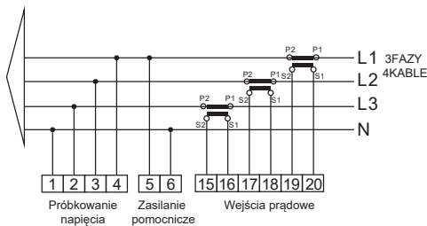
Rys. 7.13 Licznik Eastron
